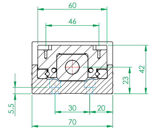
剖面圖 K-K
