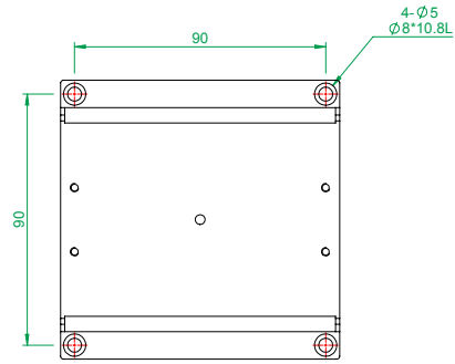
MX(Y)100-S系列 底座安裝孔尺寸
