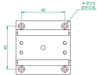
MX(Y)50-S系列 底座安裝孔尺寸
