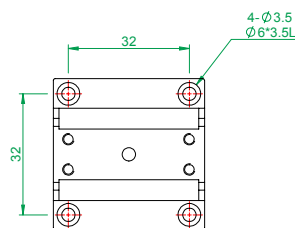
MX(Y)40-S系列 底座安裝孔尺寸
