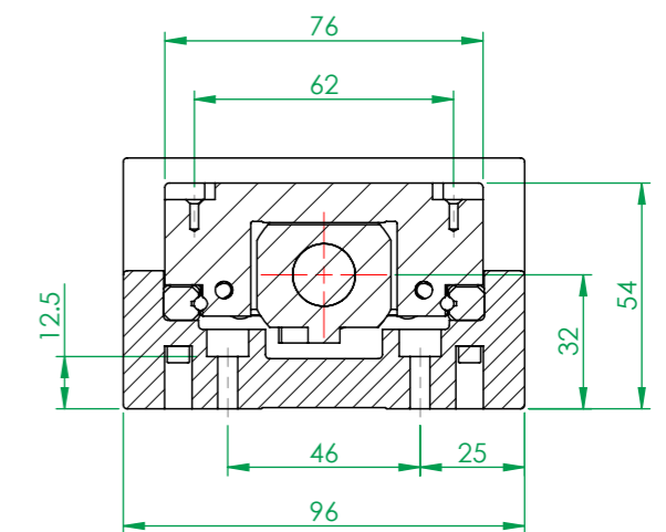
剖面圖 K-K
