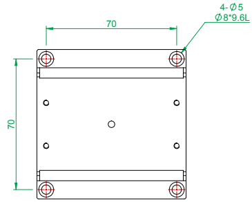
MX(Y)80-S系列 底座安裝孔尺寸
